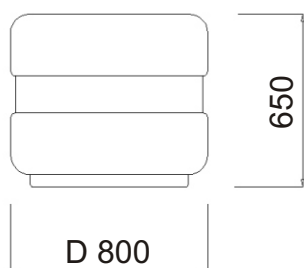
Bočný nárys
